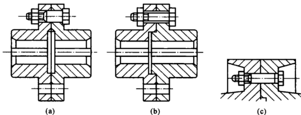
图 9-2 凸缘联轴器
